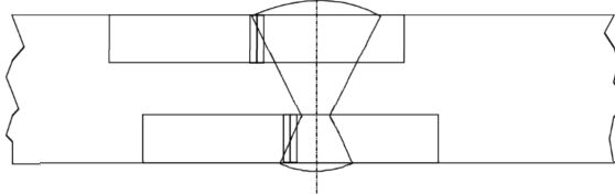
Zona de alteración debida a la soldadura
